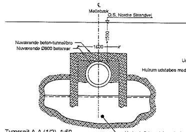
Tværsnit A-A (1/2), 1:50 Eksisterende forhold
