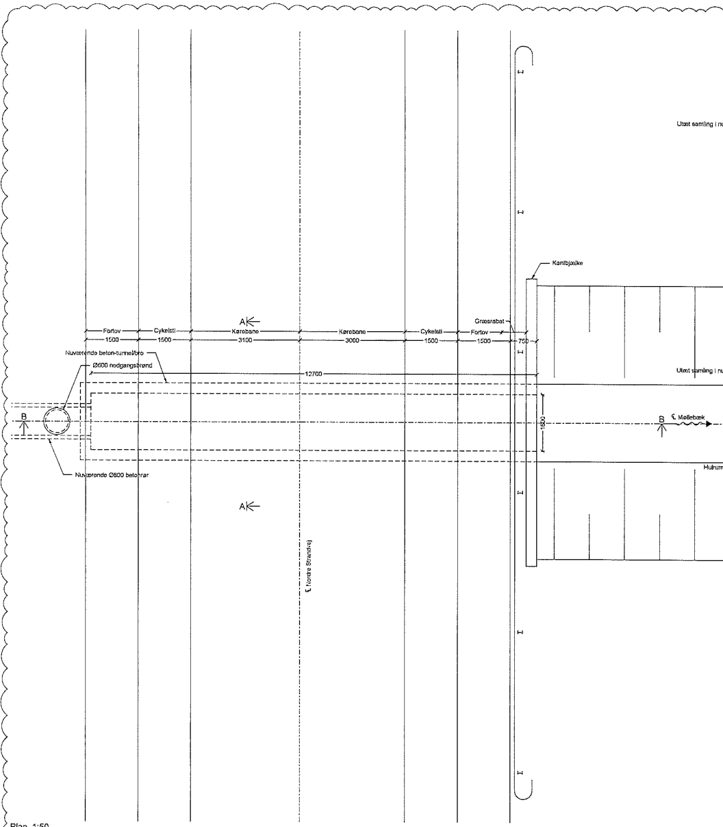
Plan, 1:50 Nordre Strandvej, U.F. af Møllebæk
