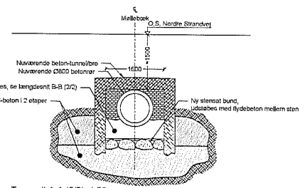
Tværsnit A-A (2/2), 1:50 Reparationsarbejder
