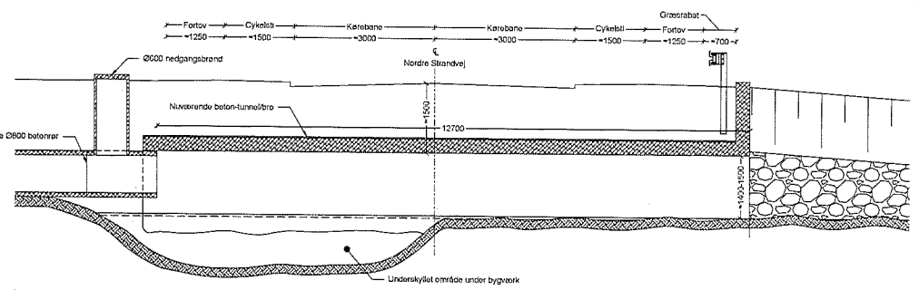
Længdesnit B-B (1/2), 1:50 Eksisterende forhold
