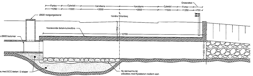
Længdesnit B-B (2/2), 1:50 Reparationsarbejder
