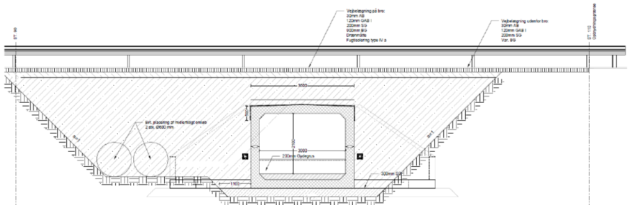
Princip for udgravning og midlertidig gennemførelse af vandføring.
